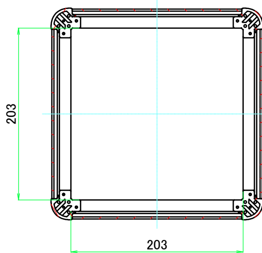
C-C ( 1 : 4.5 )
